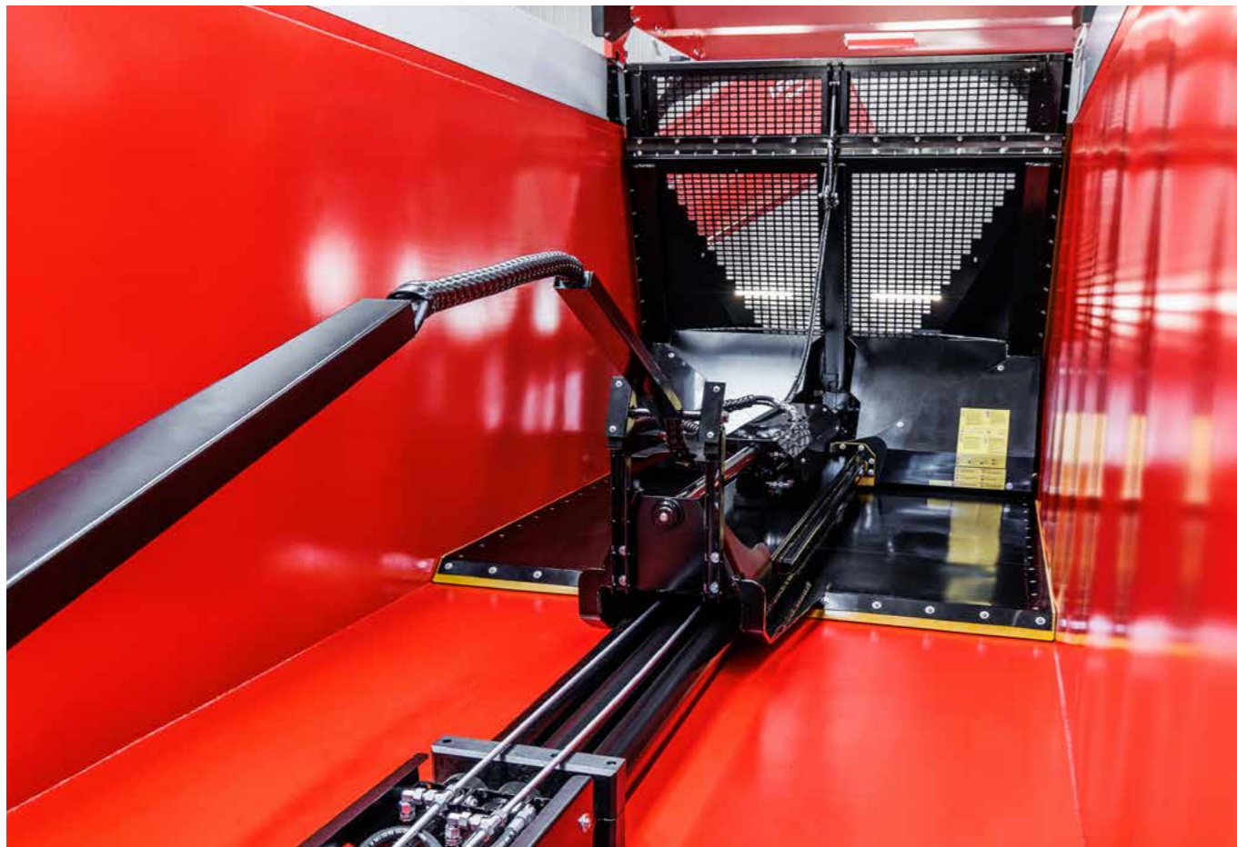
Beim Abschiebevorgang bewegen fünf Hydraulikzylinder den Schild gleichmäßig zum Fahrzeugheck. Das Schiebeschild ist im Ruhezustand in der Fahrzeugfront zusammengeklappt, somit verliert die Wanne kaum an Volumen.
